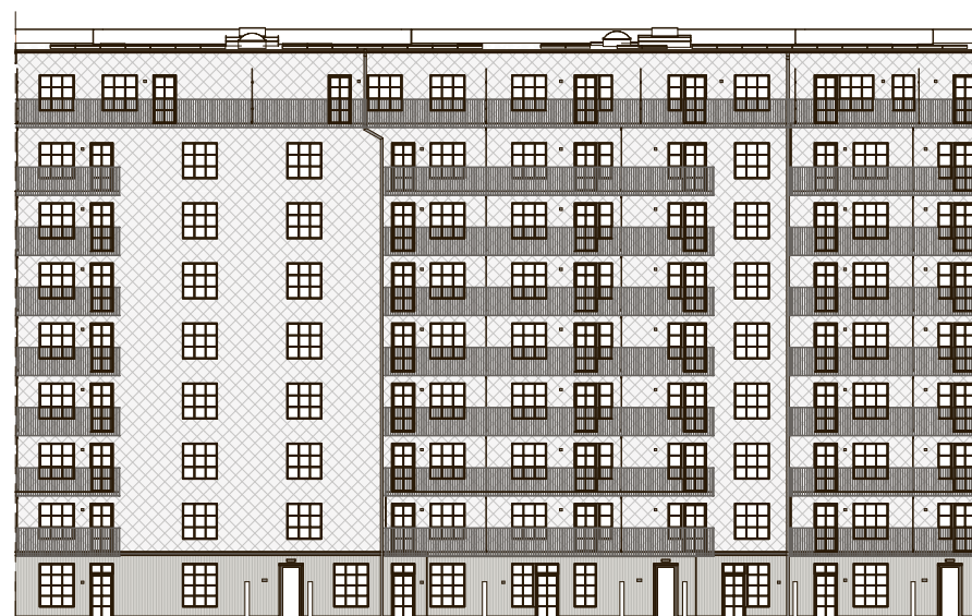
GÅRDSFASAD MOT SÖDER
