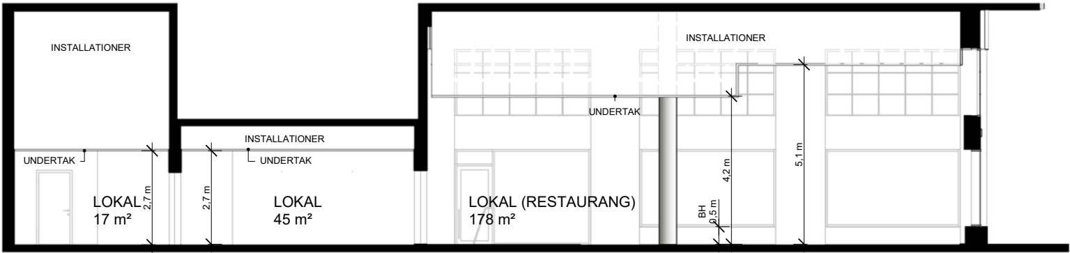
SEKTION A-A
