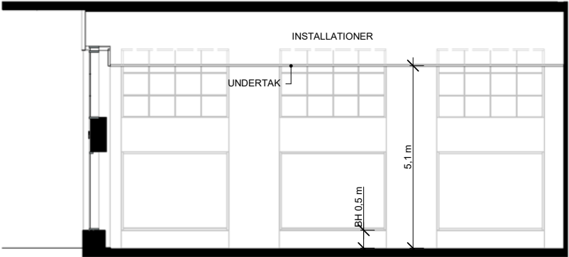
SEKTION B-B
