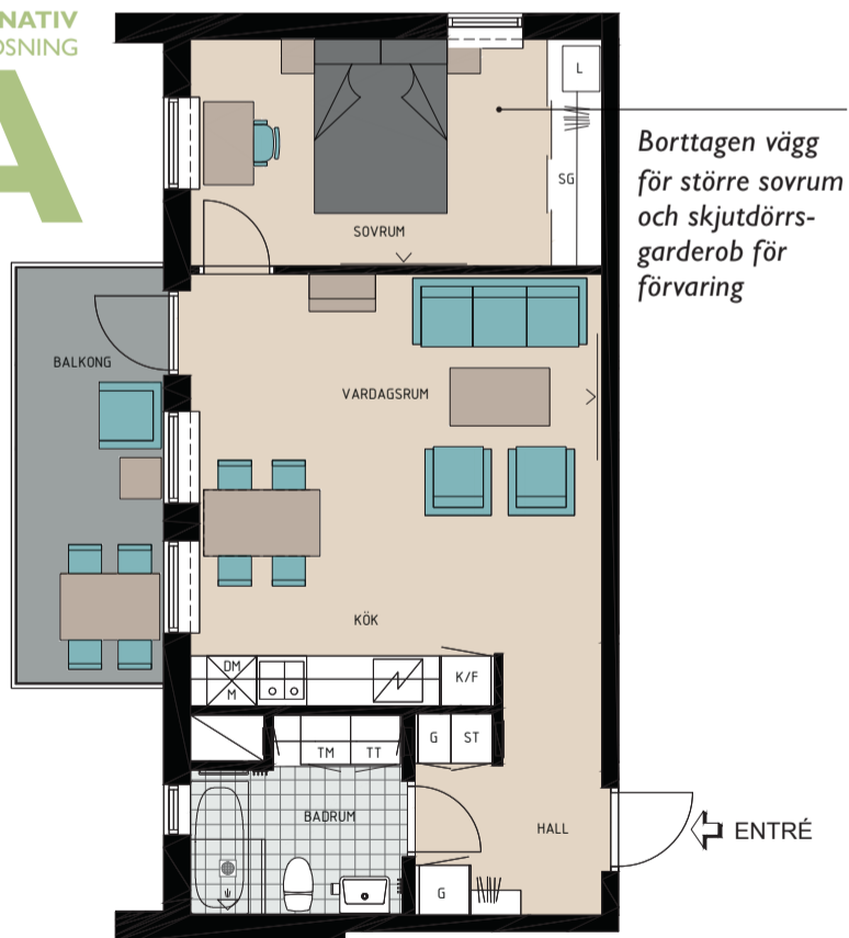
ALTERNATIV PLANLÖSNING
