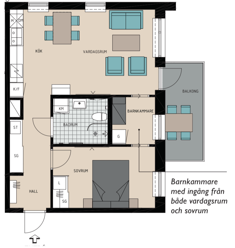
ALTERNATIV PLANLÖSNING
