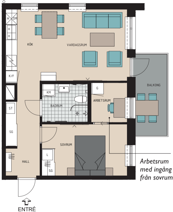
ALTERNATIV PLANLÖSNING
